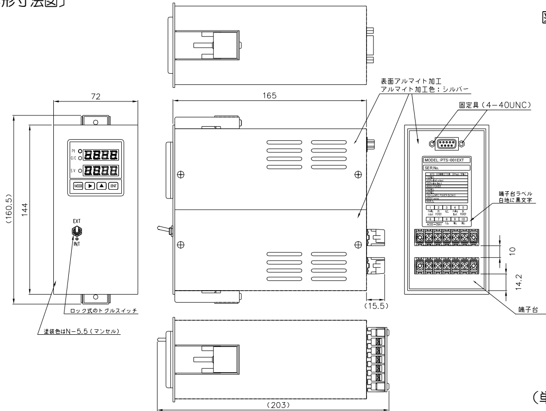
〔外形寸法図〕
